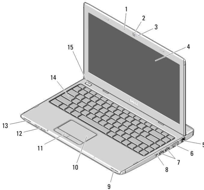
Kuva 1. Näkymä edestä
